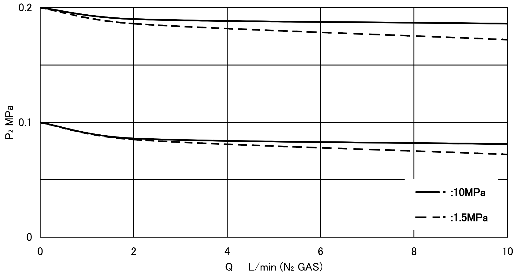
S-LABO- 0, S1, B1sr P 2 -Q (0.3MPa計) 特性
